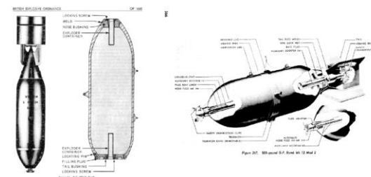
500 LB M.C. & 500 LB USA BOMBS
