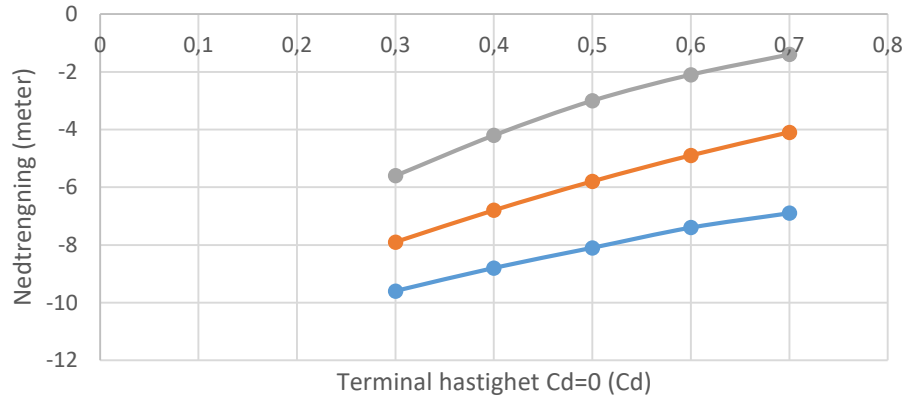
Dybde nedtrengning silt - Dropphøyde 12000 fot
